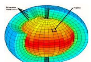
4D-EnVar AROME
